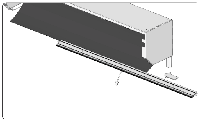
14. Rozwinąć siatkę i nasunąć na nią listwę dolną.
