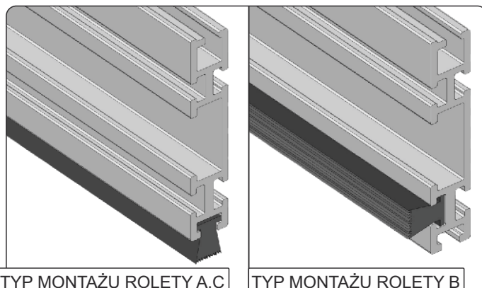
16. Do listwy dolnej moskitiery stosować uszczelkę szczotkową o wymiarach: 5,3x14mm.
